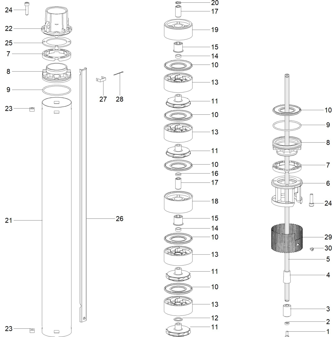
Pump end IDROSOM 22/250
