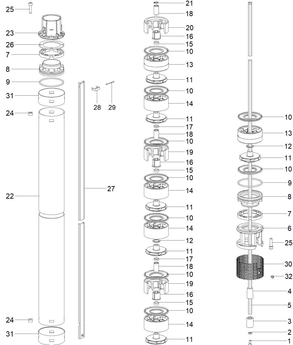
Pump end IDROSOM 30/250
