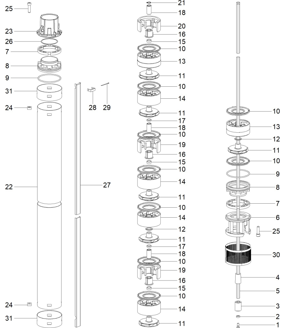
Pump end IDROSOM 31/180
