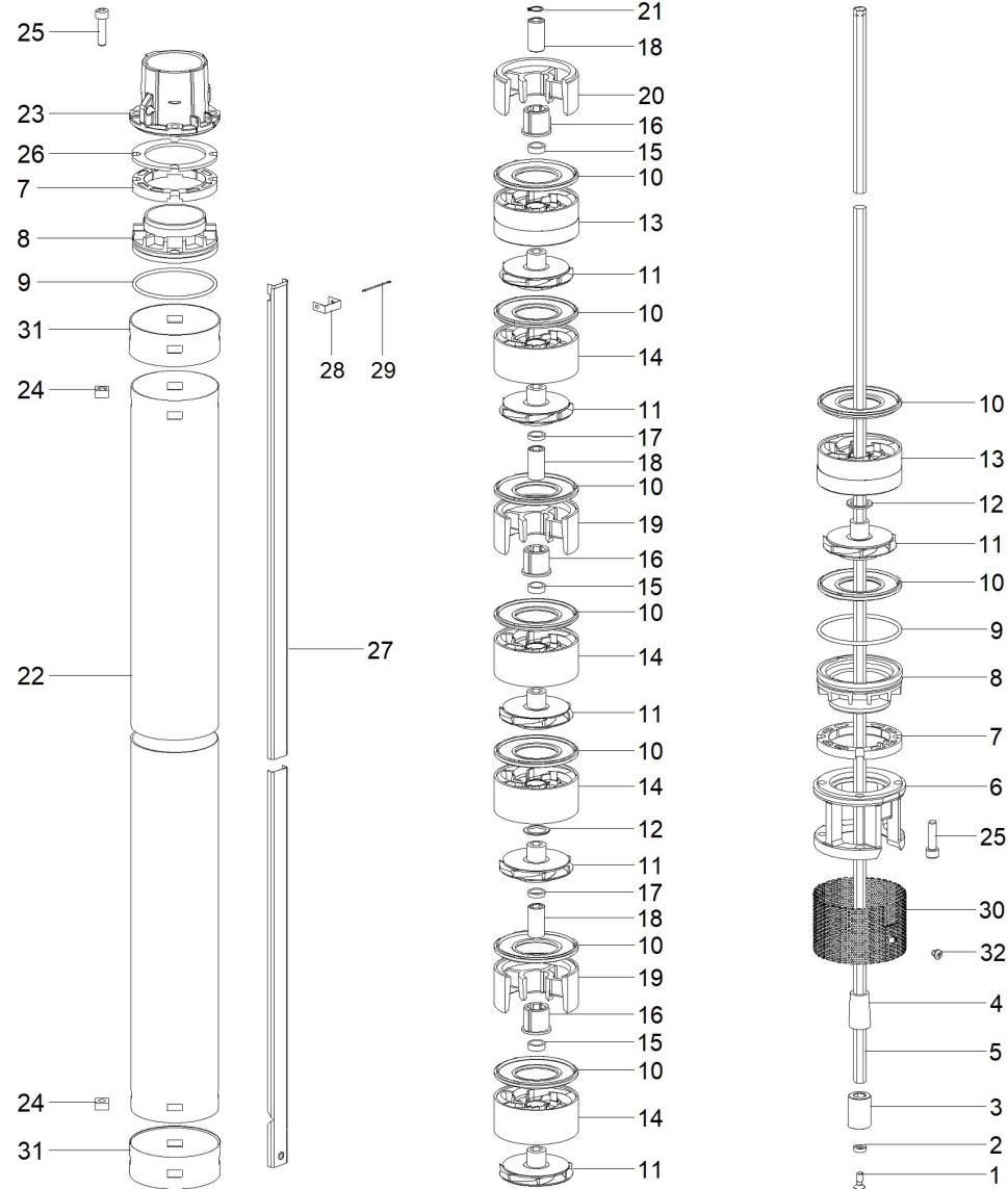
Pump end IDROSOM 40/250
