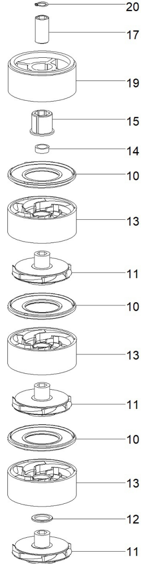
Pump end IDROSOM 8/250
