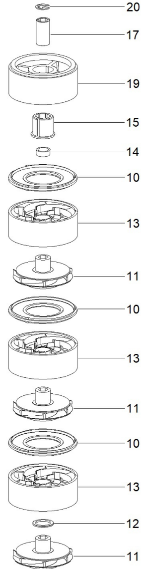
Pump end IDROSOM 9/180
