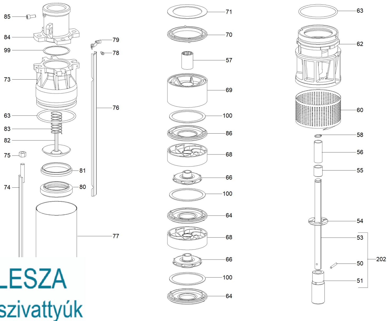
Parte pompa 6" IDROSAND 6/ 230
